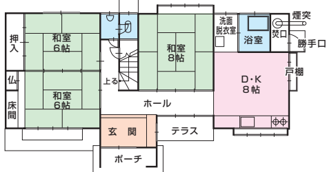
1F 平面図
