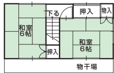
2F 平面図
