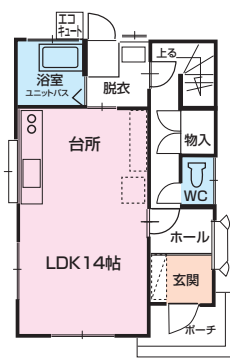
1F 平面図
